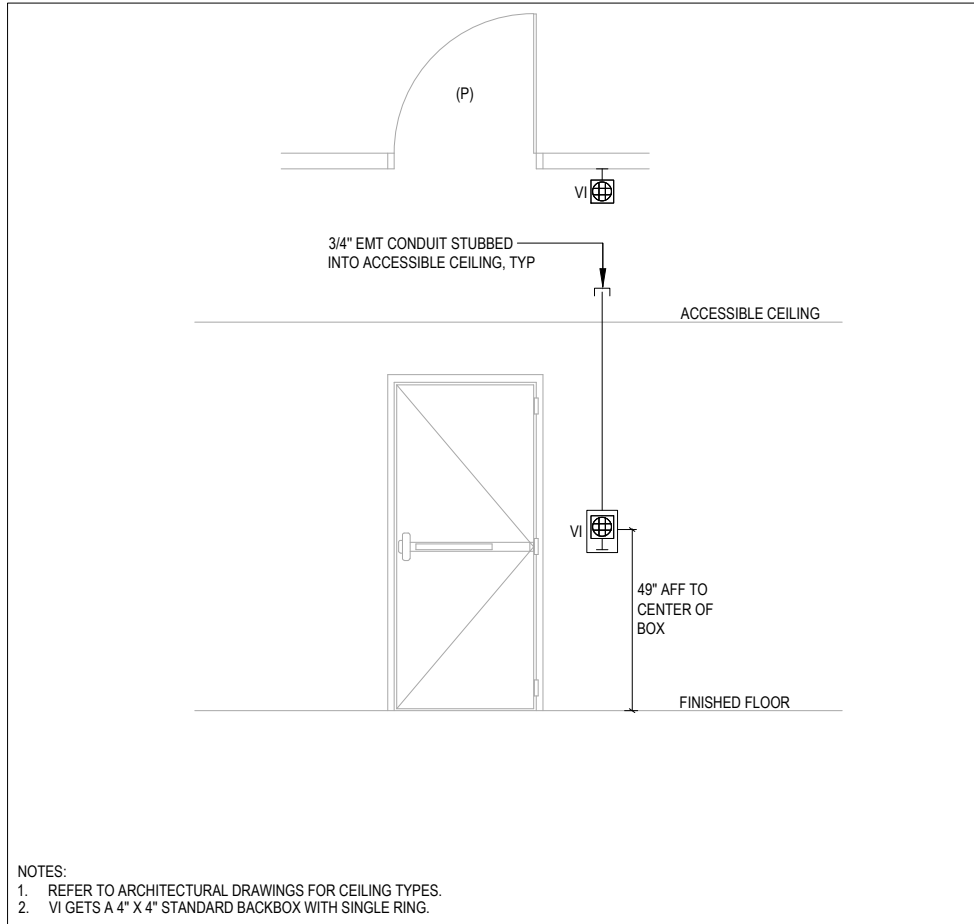
3 IP VIDEO INTERCOM SCALE: NONE
